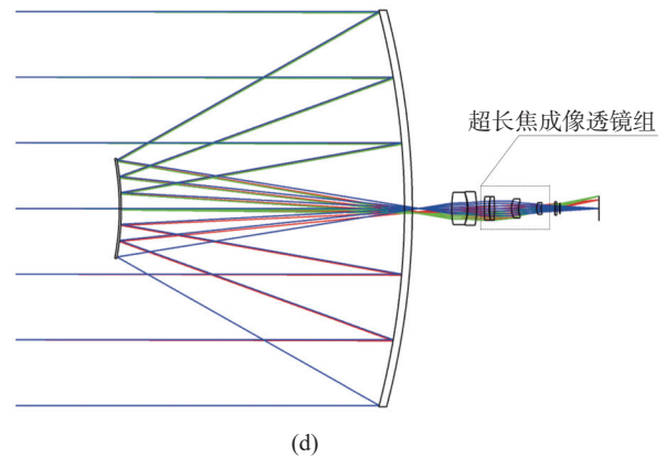
图 2 不同情况下的光学系统结构图。(a)短焦;(b)中焦;(c)长焦;(d)超长焦
