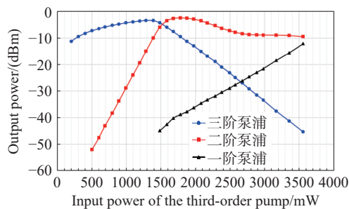
图 6 仅三阶泵浦光输入时,各阶泵浦光功率随三阶泵浦光输入功率变化
