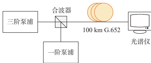
图 3 仅泵浦作用时的实验装置
