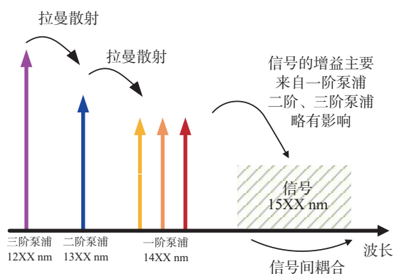
图 1 三阶拉曼光纤放大器工作原理
