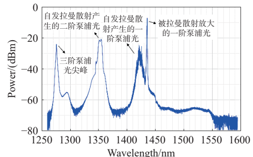
图 5 输入一阶和三阶泵浦光时输出端光谱
