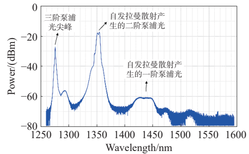
图 4 仅输入三阶泵浦光时输出端光谱
