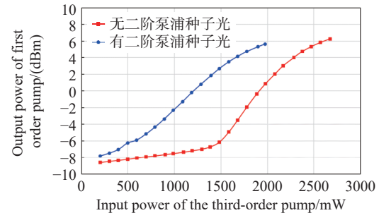
图 8 二阶泵浦种子光对一阶泵浦光输出功率的影响
