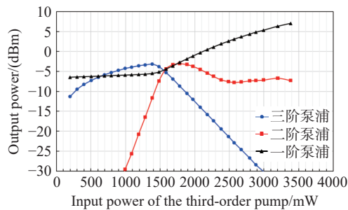
图 7 一阶+三阶泵浦光输入时,各阶泵浦光功率随三阶泵浦光输入功率变化
