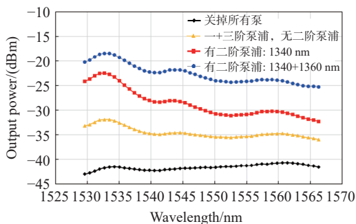
图 11 输出信号功率比较
