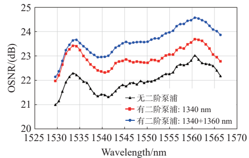
图 12 输出信号光信噪比较
