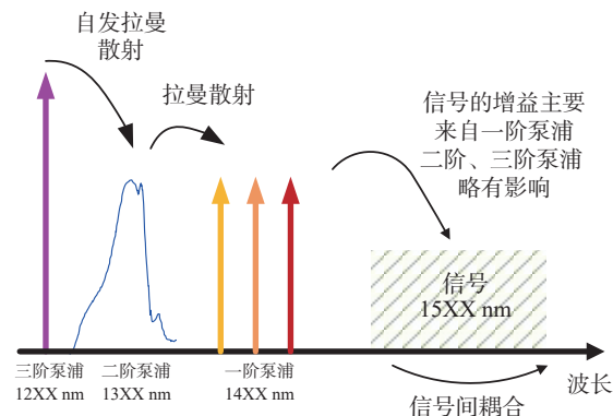
图 2 无二阶泵浦种子光时三阶拉曼光纤放大器工作原理
