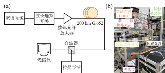
图 9 实验装置: (a) 框图; (b) 实物图
