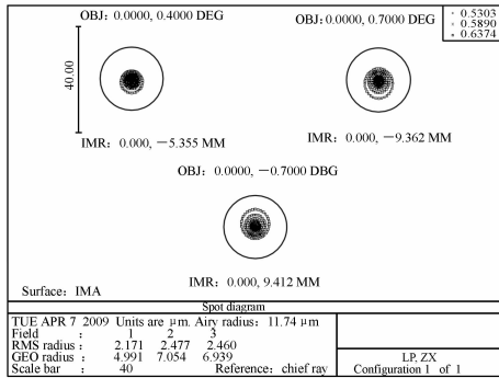
图 4 日冕系统点列图
