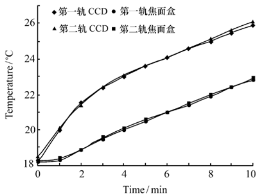
图9 遥感器工作时 CCD 及焦面盒温度曲线
